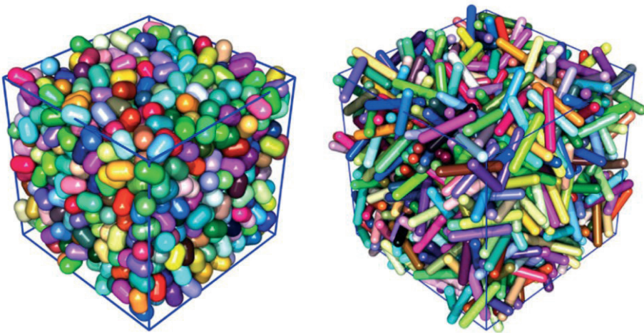
Rys. 2.35. Złoża utworzone z sferocylinдры o różnym wydłużeniu: a – w = 0,5 ; \varphi = 0,725 , b – w = 5 ; \varphi = 0,561
