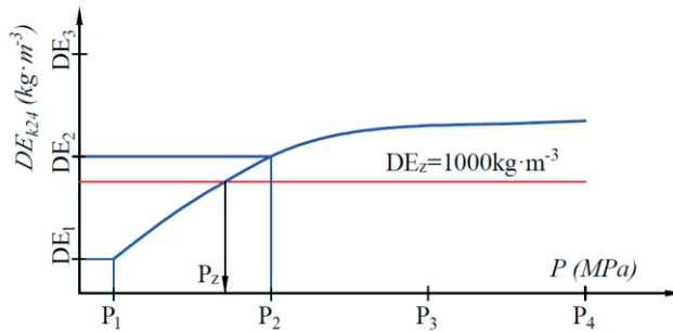
Rys. 4.13. Graficzny sposób wyznaczania zagęszczalności progowej
