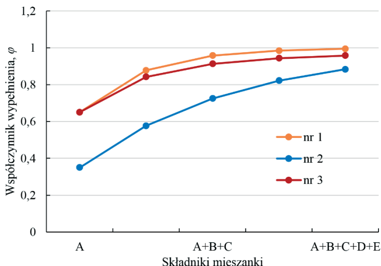
Rys. 4.20. Przebieg zmian współczynnika wypełnienia \varphi dla mieszanki utworzonych z pięciu frakcji A, B, C, D, E. Krzywa nr 1 \varphi = 0,65 ; nr 2 \varphi = 0,35 ; nr 3 \varphi w zakresie 0,25 – 0,65
