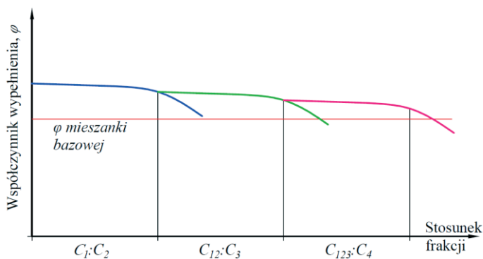
Rys. 4.23. Zasada autorskiej metody iteracyjnego komponowania składu ziarnowego mieszanki biomasowej
