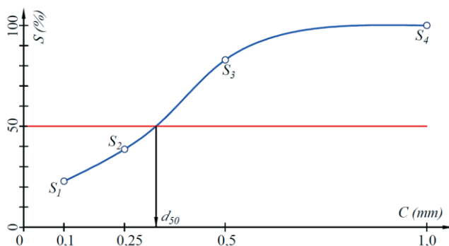
Rys. 4.4. Przykład wykresu skumulowanego składu ziarnowego wraz ze sposobem graficznego wyznaczania d_{50}
