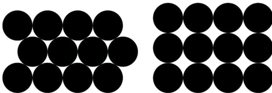
Rys. 2.34. Regularny układ dysków na płaszczyźnie: a – heksagonalny, b – kubiczny.
