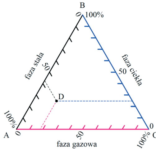
Rys. 2.24. Diagram składu fazowego
