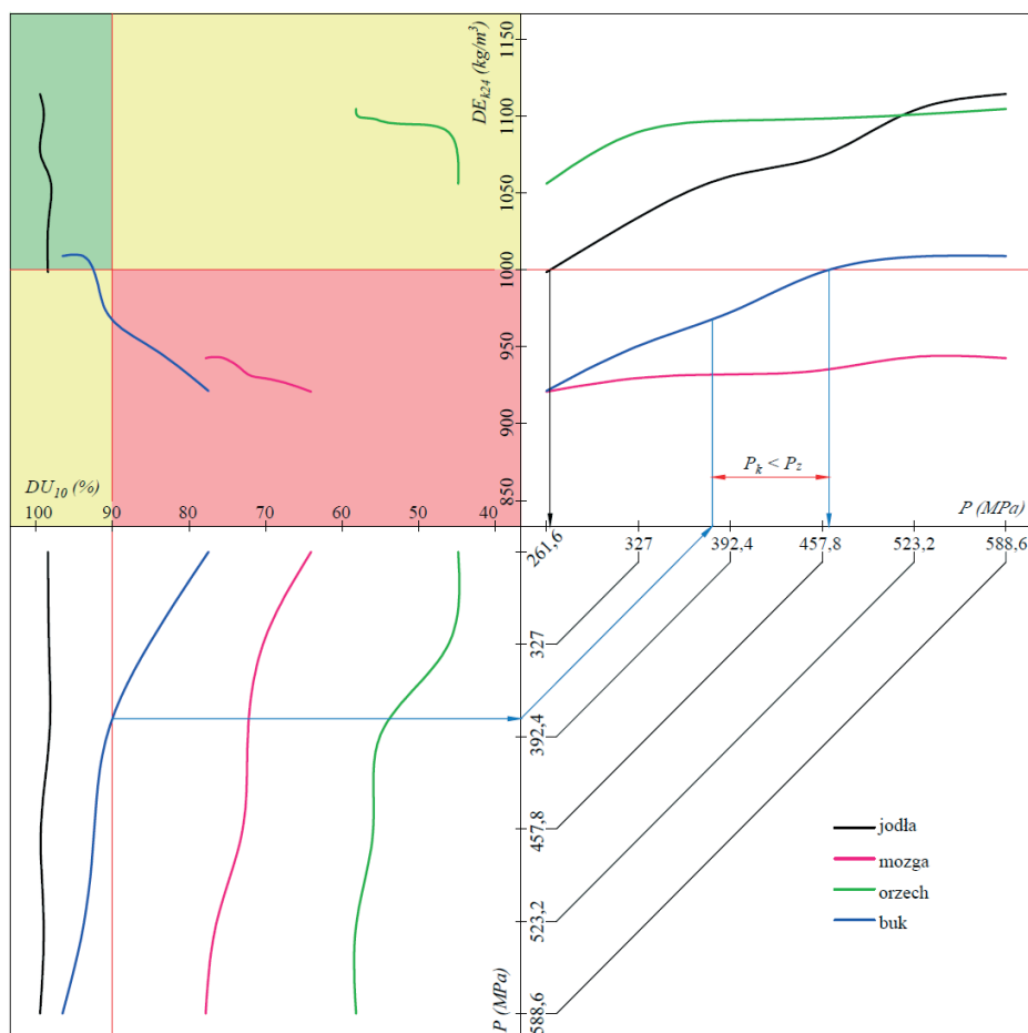
Rys. 5.15. Nomogram zagęszczalności i kompaktowalności biomasy jodły, mozgi, buka i łupin orzecha
