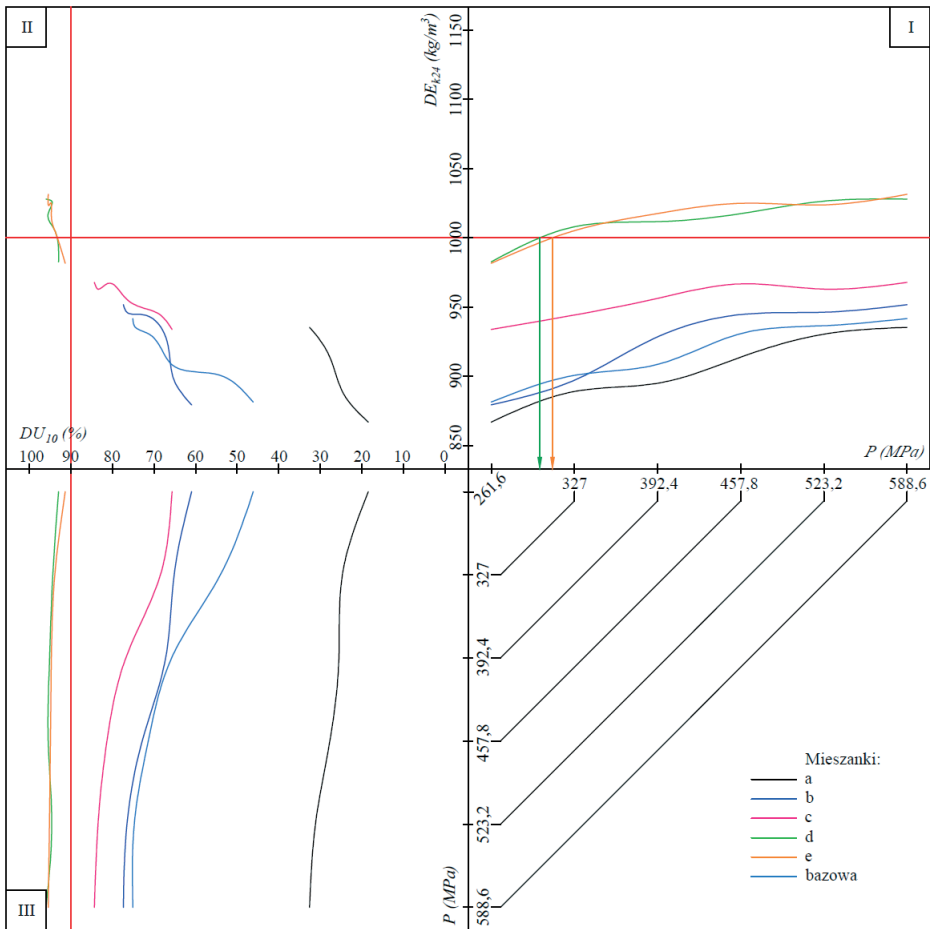
Rys. 5.24. Nomogram mieszanek biomasy wierzy
