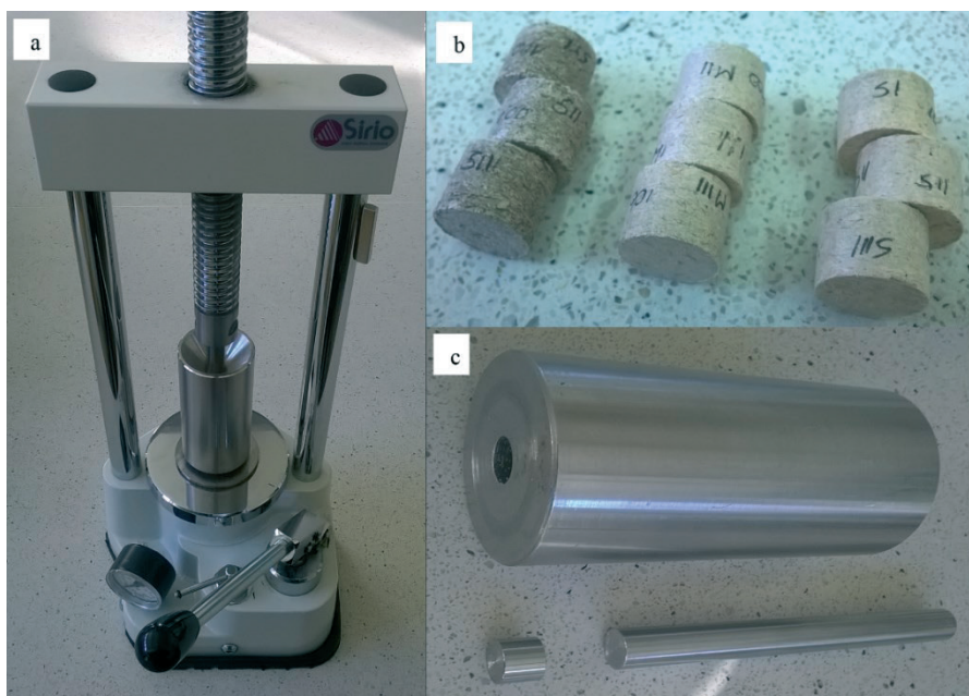
Rys. 4.7. Stanowisko zagęszczania próbek: a – prasa hydrauliczna, b – przykładowe granule, c – zestaw zagęszczający tuleja – tłok – przeciwtłok
