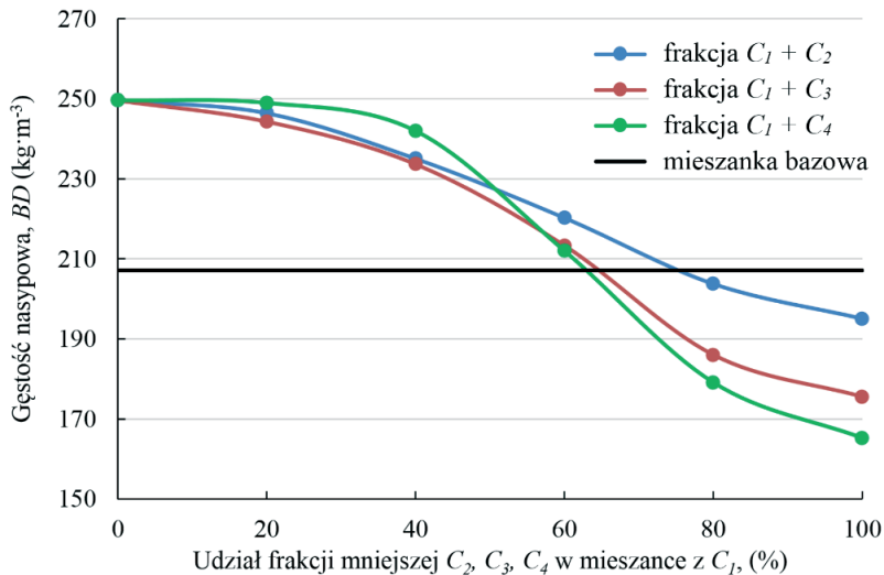
Rys 5.17. Krzywe przebiegu zmian gęstości nasypowej BD mieszanek dwóch frakcji wymiarowych biomasy mózgi
