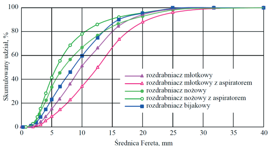
Rys. 2.32. Porównanie skumulowanych składów ziarnowych próbki siana rozdrabnianego za pomocą różnych urządzeń rozdrabniających wyposażonych w sito o średnicy otworów 4 mm
