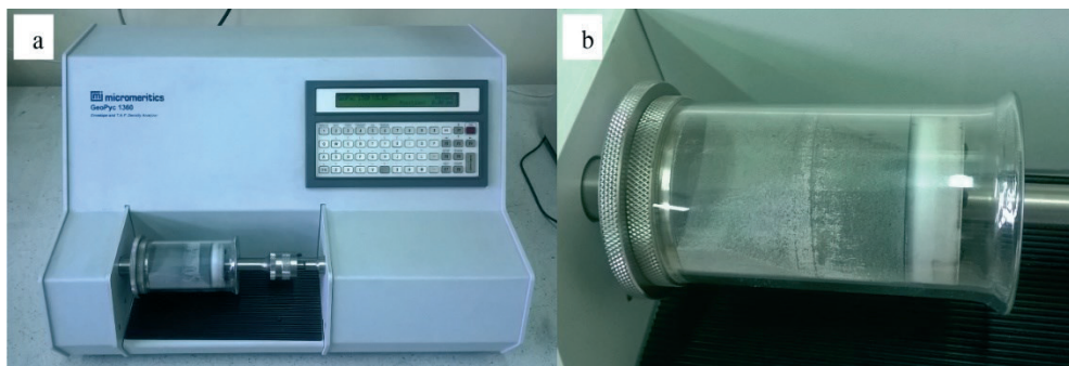
Rys. 4.2. Piknometr quasieczystowy GeoPyc 1360: a – widok ogólny, b – cylinder pomiarowy
