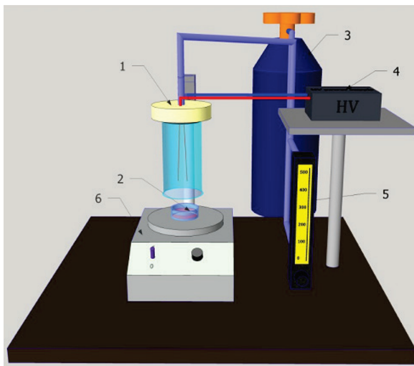
Rys. 2. Schemat stanowiska badawczego z reaktorem plazmowym GAD 1 – GAD; 2 – próbka; 3 – zasilanie gazem; 4 – zasilanie; 5 – przeływomierz; 6 – mieszkadło magnetyczne
