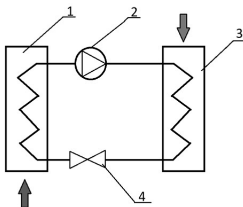
Rysunek 3.7. Widok i schemat budowy pompy ciepła. (1) parownik; (2) sprężarka; (3) skraplacz; (4) zawór rozprężny (R. Szulc)
