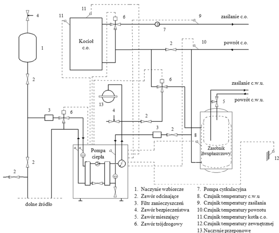
Rys. 5.4. Przykład węzła ciepłego (Oprac. Rzeźnik W., Rzeźnik I.)
