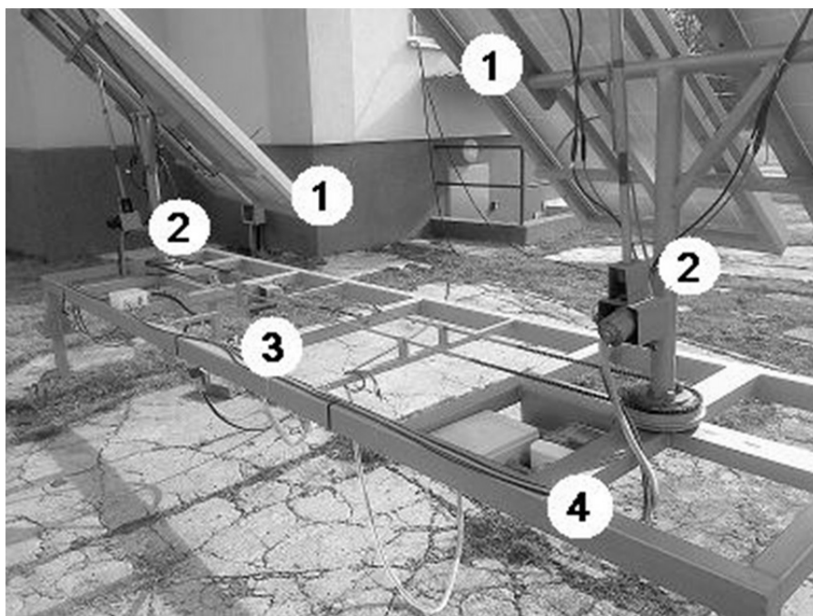
Rysunek 6.8. Mechanizm heliostatyczny: 1) moduły fotowoltaiczne 2) silowniki zmieniające kąt nachylenia modułów 3) silownik umożliwiający obrót modułów wokół osi pionowej 4) układ automatycznego sterowania silownikami na podstawie sygnałów z czujnika promieniowania, z możliwością sterowania manualnego (Foto. J. Lenarczyk)
