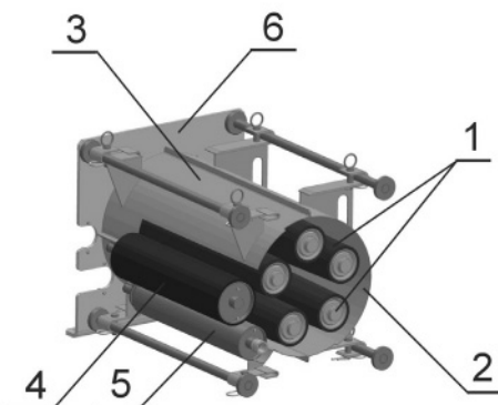
Rysunek 1.3. Schemat komory brykietującej urządzenia brykietującego niepociętą biomasę metodą zwijania. (1) komora brykietowania, (2) dolna osłona zespołu brykietującego, (3) górna osłona zespołu brykietującego, (4) górny walec wstępnego zagęszczania, (5) dolny walec wstępnego zagęszczania, (6) płyta boczna korpusu zespołu brykietującego
