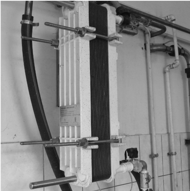
Rysunek 3.1. Płytowy wymiennik ciepła do mleka (Źródło: R. Szulc)
