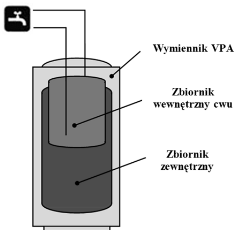
Rysunek 5.5. Budowa zasobnika dwupłaszczowego typu VPA (Oprac. Rzeźnik W., Rzeźnik I.)
