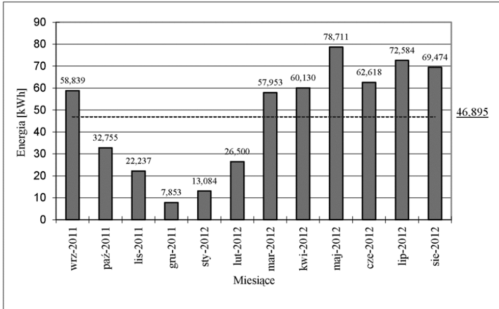
Rysunek 6.11. Ilość uzyskanej energii elektrycznej przez panele fotowoltaiczne o łącznej mocy szczytowej 668W w okresie pomiarowym (kWh); wartość podkreślona – średnia arytm.
