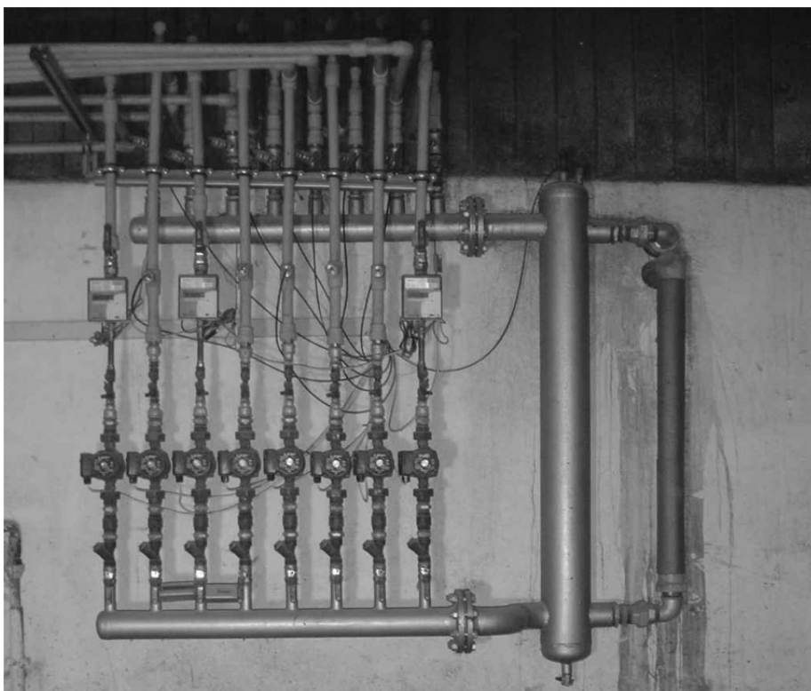
Rysunek 5.3. Sprzęgło hydrauliczne z rozdzielaczem w badanej tuczarni
