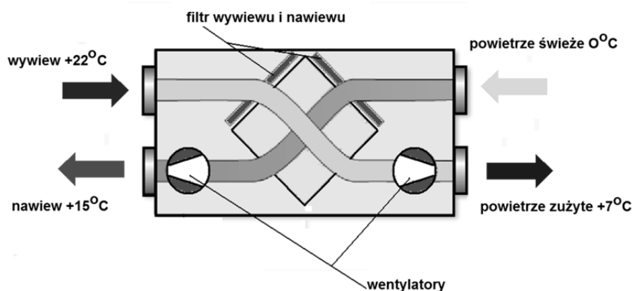
Rysunek 3.6. Zasada działania wymiennika krzyżowego ( R. Szulc)
