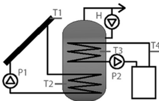
Rysunek 3.14. Zasada ładowania zasobnika CWU energią z kolektora słonecznego oraz możliwością dogrzewania zasobnika z zewnętrznego źródła ciepła (Źródło: Katalog BIAWAR NIBE 2010)
